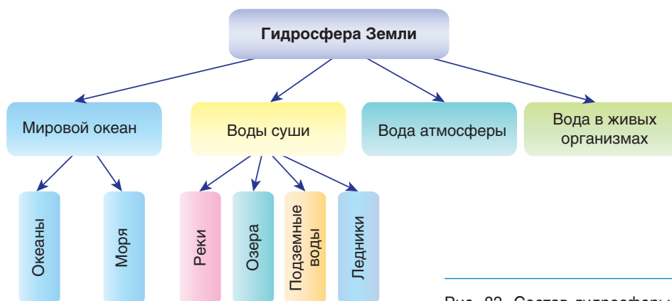
Рис. 83. Состав гидросферы
